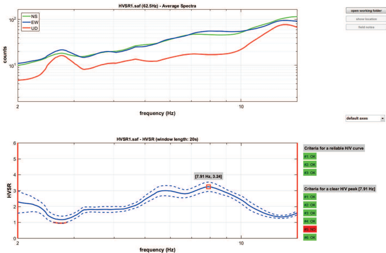
Figura 23: Dati HVSr, nella misura 1 a 7.91 Hz è stato individuato un picco di 3.24 Nella colonna di destra possiamo vedere la verifica dei criteri di ammissibilità del progetto SESAME
