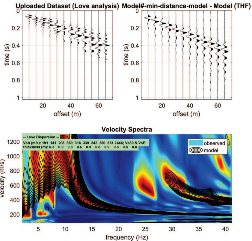
Figura 56: Modello distanza minima in full velocity spectral per le onde di Love
