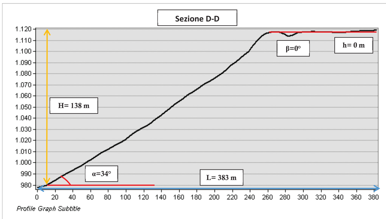
Figura 10: Ubicazione e sezione DD per scenario Z3a
