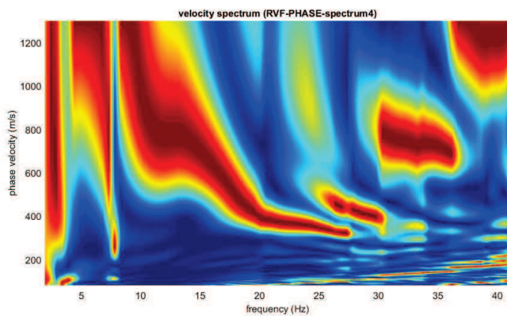
Figura 50: Spetto di velocità, Dataset Onde Rayleigh componente radiale (RVF)
