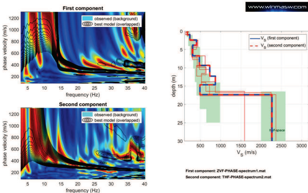
Figura 39: Inversione congiunta Full velocity spectral Rayleigh e Love
