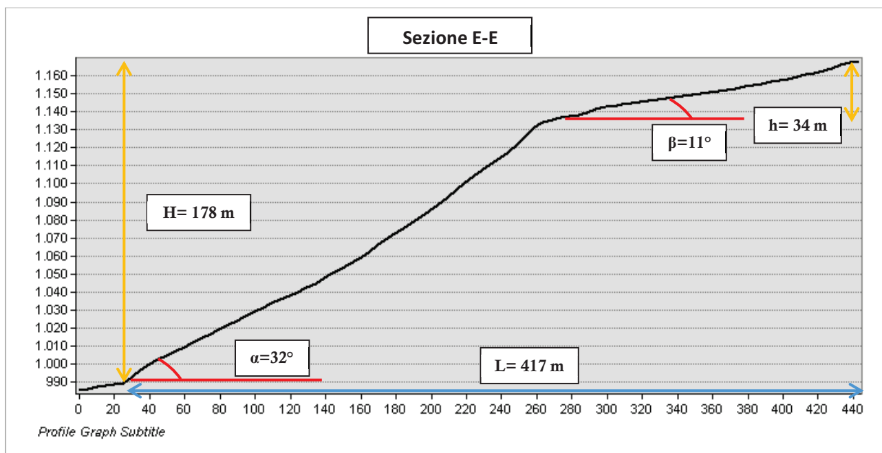
Figura 11: Ubicazione e sezione EE per scenario Z3a
