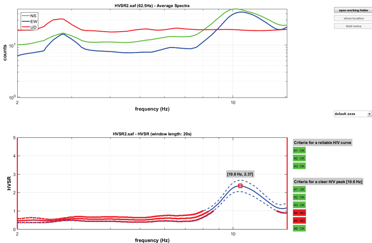
Figura 68: Dati HVS2, nella misura 2 a 10.6 Hz è stato individuato un picco di 2.37 Nella colonna di destra possiamo vedere la verifica dei criteri di ammissibilità del progetto SESAME
