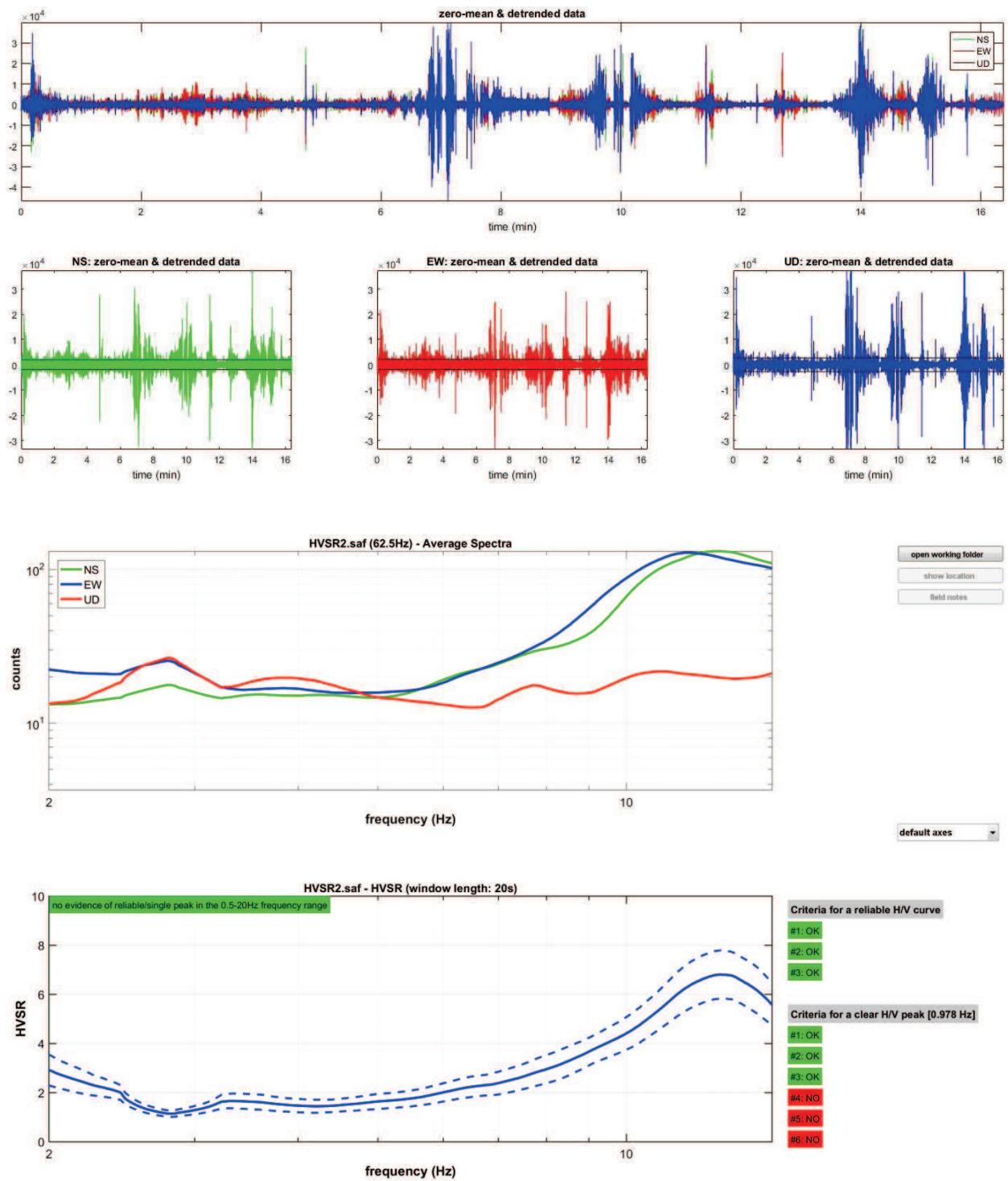
Figura 52: Dati HVSR, nella misura 1 non sono stati evidenziati picchi rappresentativi. Nella colonna di destra possiamo vedere la verifica dei criteri di ammissibilità del progetto SESAME
