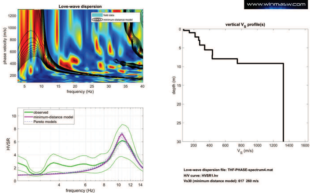
Figura 69: Analisi congiunta onde Love e HVS2 4
