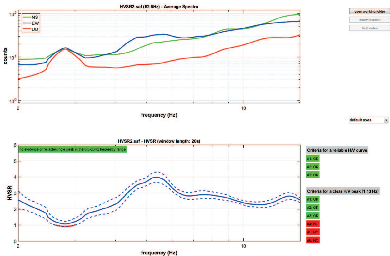
Figura 38: Dati HVS2, nella misura 2 non sono stati evidenziati picchi rappresentativi. Nella colonna di destra possiamo vedere la verifica dei criteri di ammissibilità del progetto SESAME
