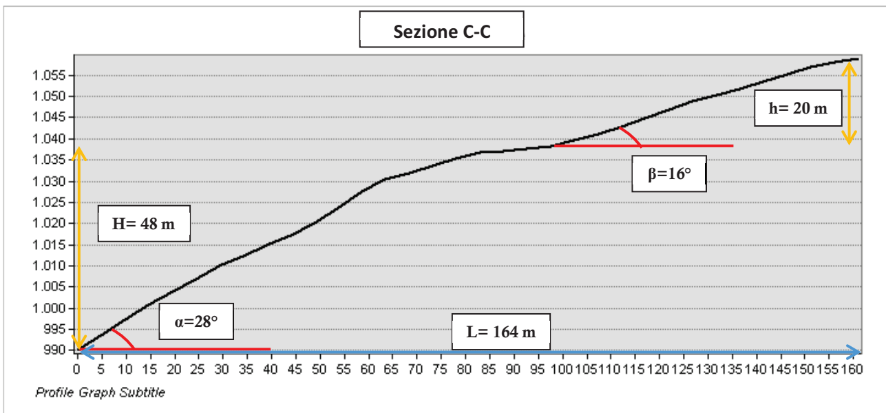
Figura 9: Ubicazione e sezione CC per scenario Z3a
