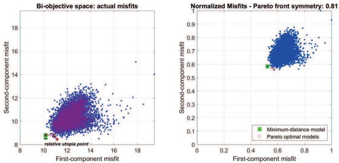
Figura 42: Diagramma distribuzione pareto ed errori attuale
