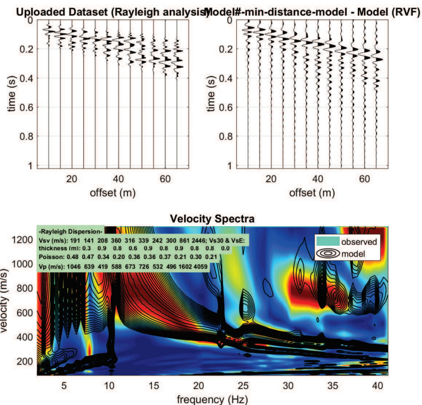
Figura 55: Modello distanza minima in full velocity spectral per le onde di Rayleigh
