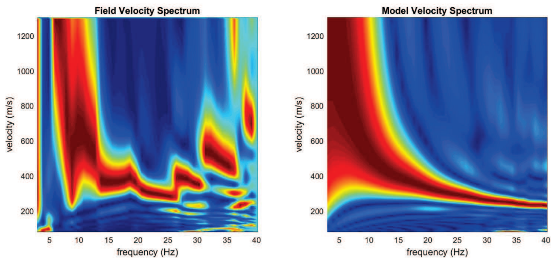
Figura 26: Modello di campo e modello sintetico
