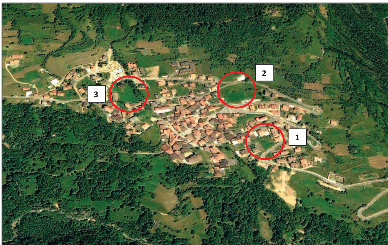
Figura 16: Ubicazione delle aree dove sono state eseguite MASW e HVSR nel Comune di Monno
