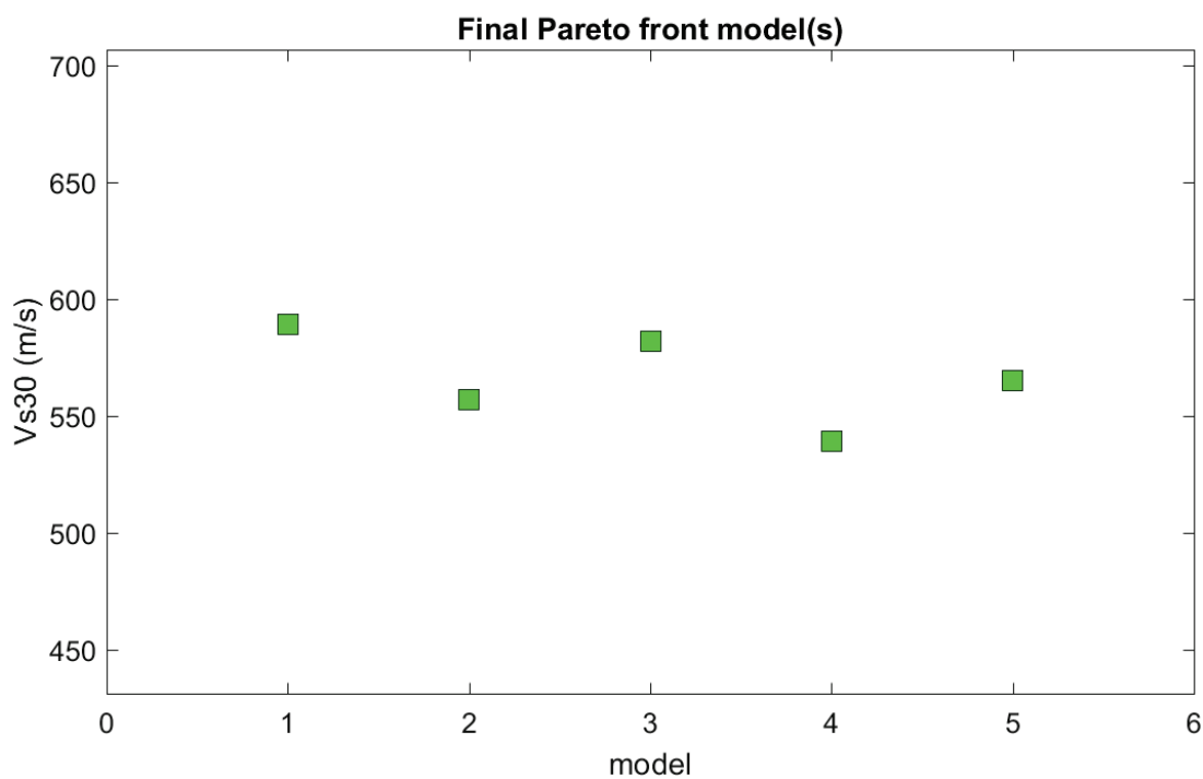
Figura 28: Distribuzione pareto Vs 30
