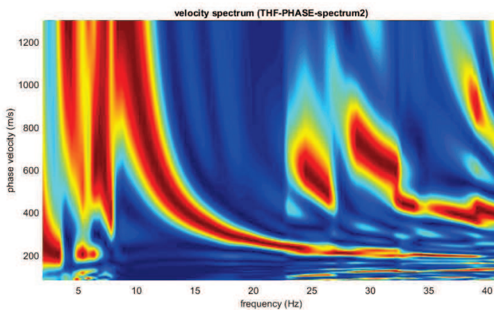
Figura 51: Spetto di velocità, Dataset Onde Love componente orizzontale (THF)
