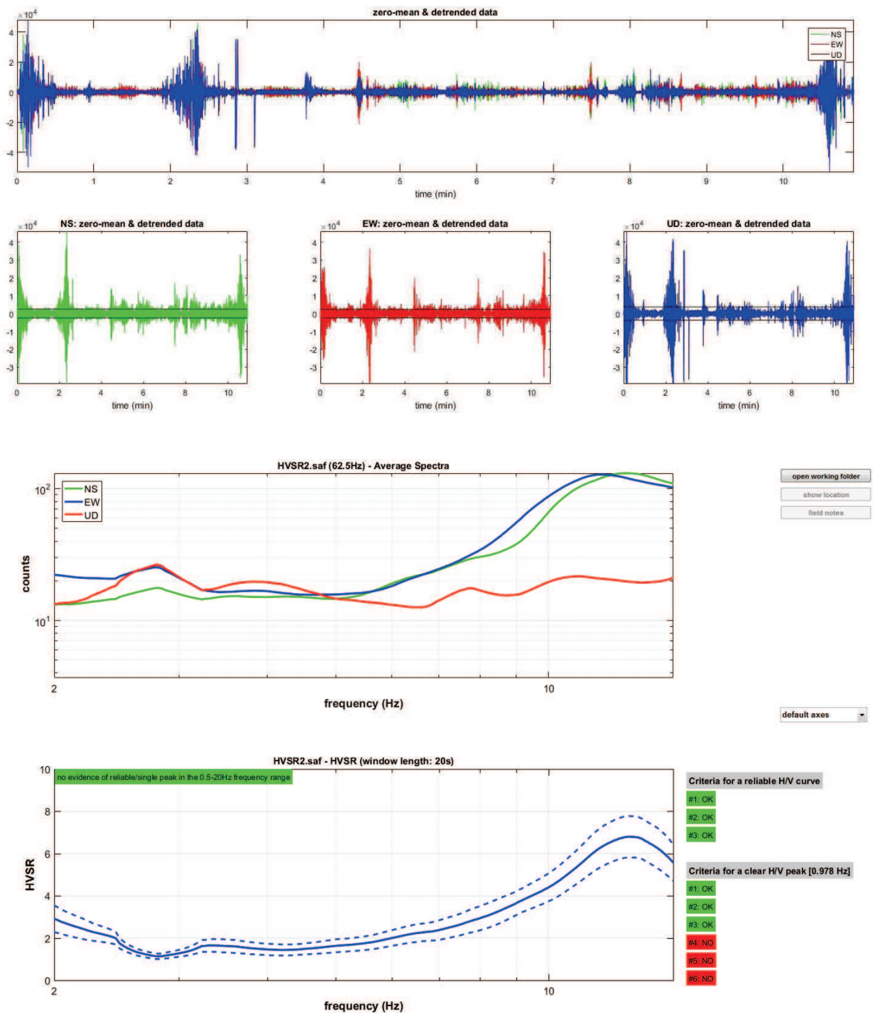
Figura 53: Dati HVSr, nella misura 2 non sono stati evidenziati picchi rappresentativi. Nella colonna di destra possiamo vedere la verifica dei criteri di ammissibilità del progetto SESAME
