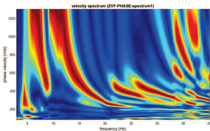
Figura 34: Spetto di velocità, Dataset Onde Rayleigh componente verticale (ZVF)
