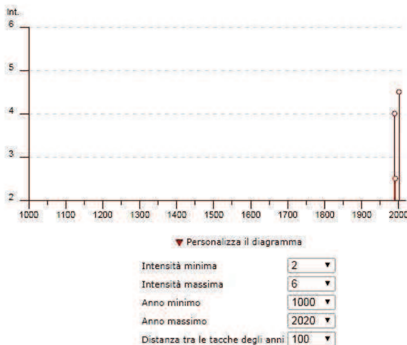
Figura 4: Database Macrosismico Italiano chiamata DBMI15
