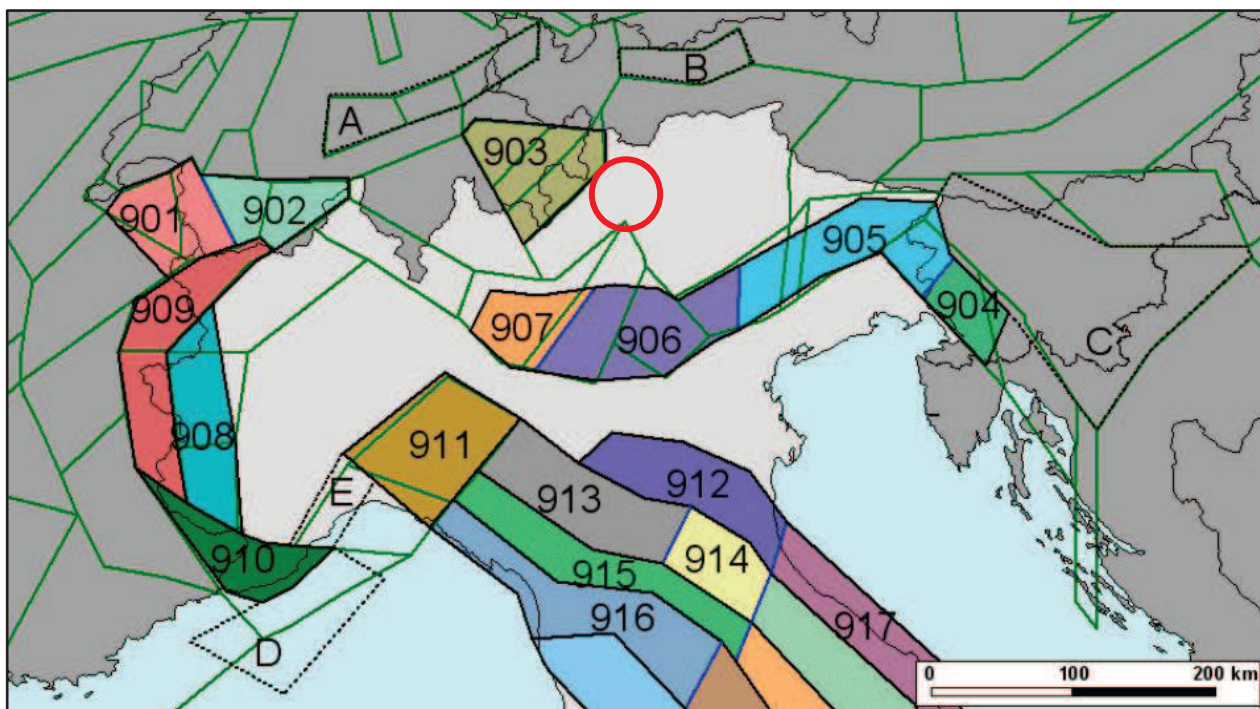
Figura 2: Stralcio della zonazione sismogenetica ZS9
