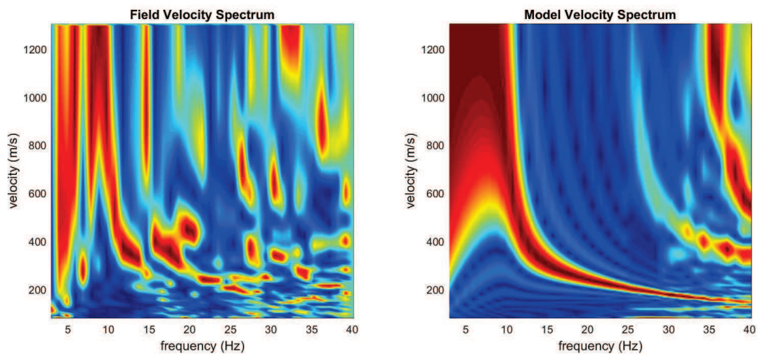
Figura 70: Modello di campo e modello sintetico
