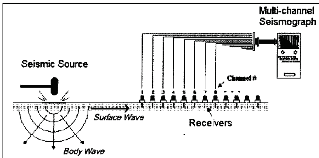
Figura 18: Schema stendimento sismico MASW
