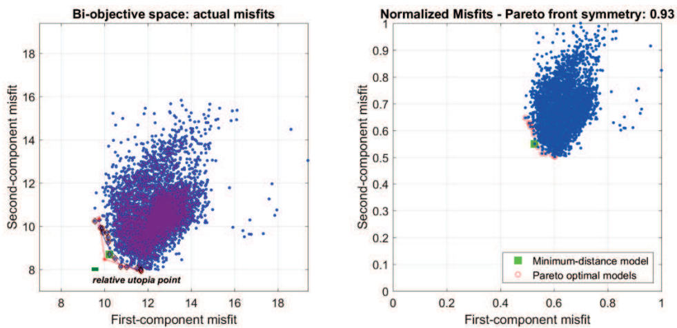
Figura 57: Diagramma distribuzione pareto ed errori attuale
