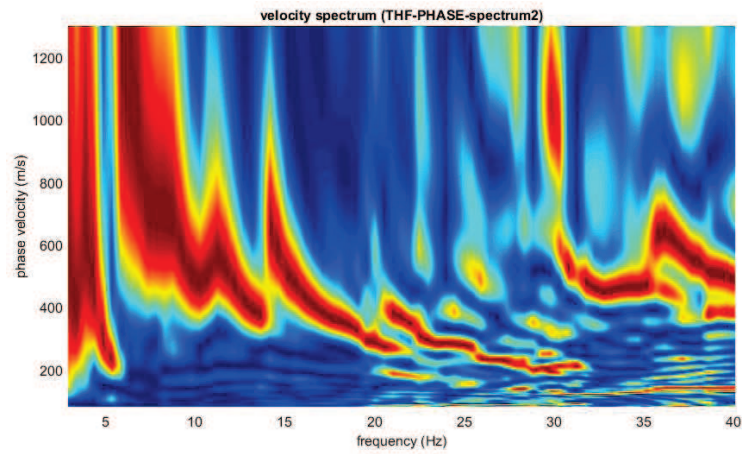
Figura 36: Spetto di velocità, Dataset Onde Love componente orizzontale (THF)
