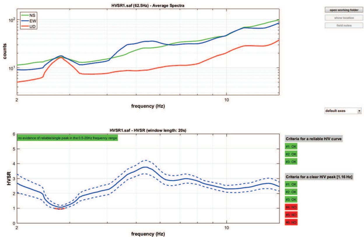
Figura 37: Dati HVS, nella misura 1 non sono stati evidenziati picchi rappresentativi. Nella colonna di destra possiamo vedere la verifica dei criteri di ammissibilità del progetto SESAME
