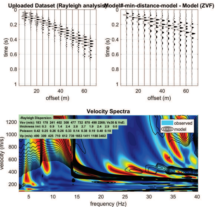
Figura 40: Modello distanza minima in full velocity spectral per le onde di Rayleigh
