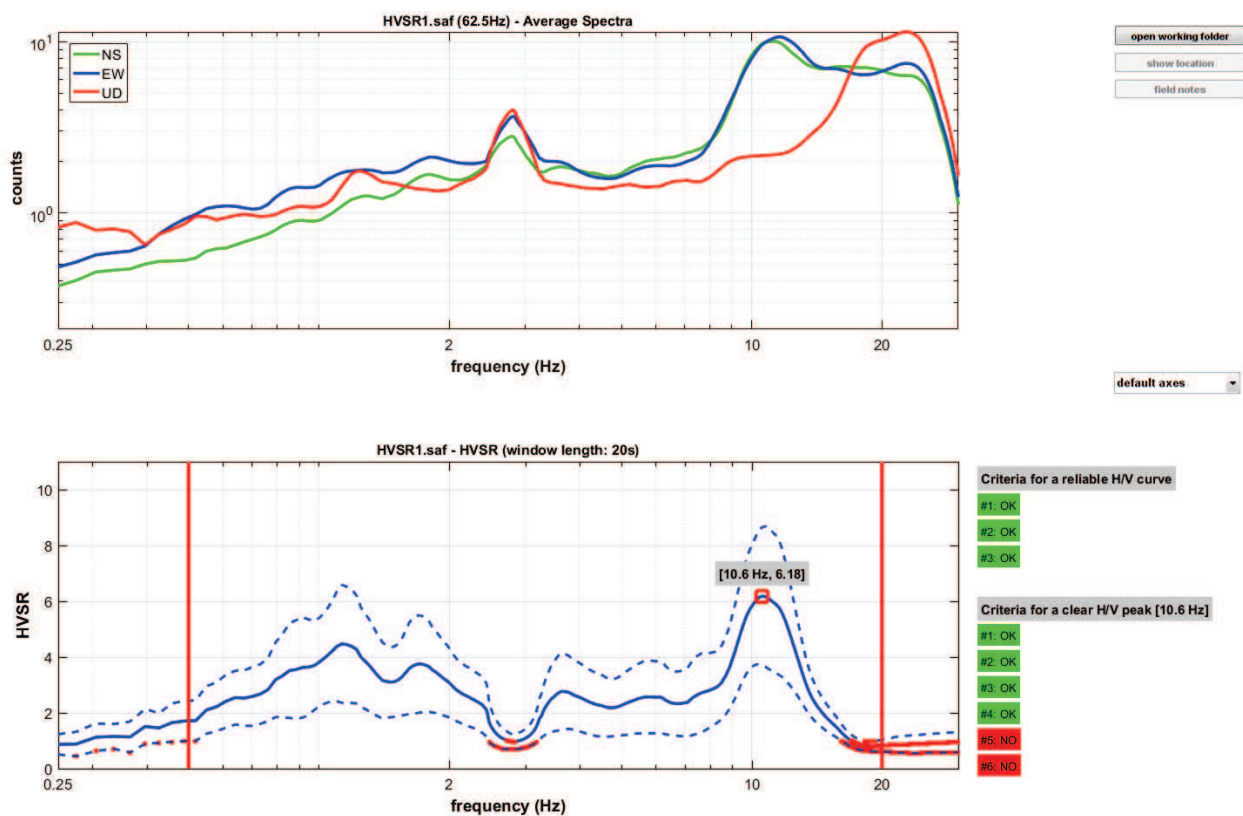
Figura 67: Dati HVSr, nella misura 1 a 10.6 Hz è stato individuato un picco di 6.18 Nella colonna di destra possiamo vedere la verifica dei criteri di ammissibilità del progetto SESAME
