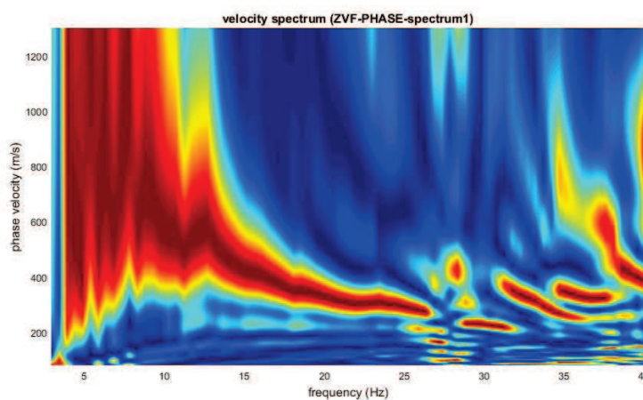
Figura 20: Spetto di velocità, Dataset Onde Rayleigh componente verticale (ZVF)
