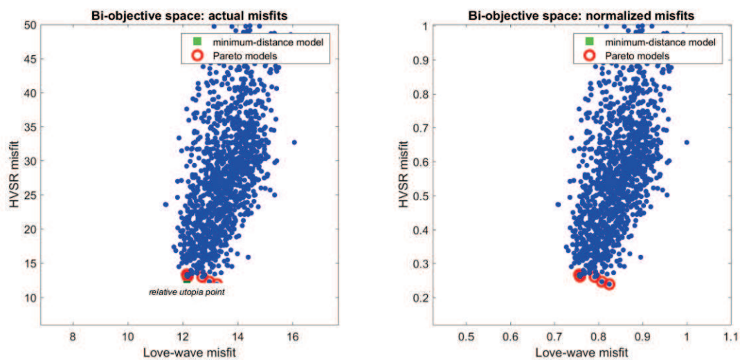
Figura 71: Grafico tra errore HVSR e Love, attuale e normalizzato
