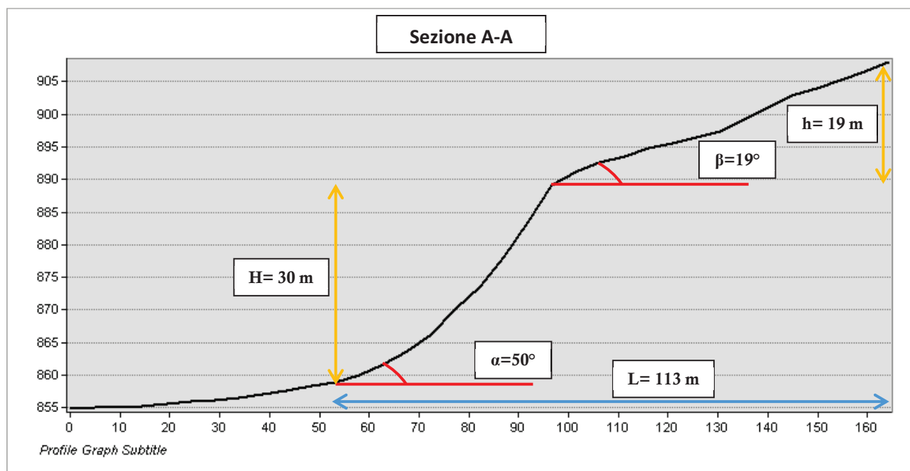
Figura 7: Ubicazione e sezione AA per scenario Z3a
