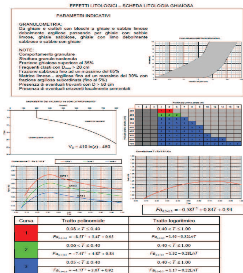
Figura 76: Scheda litologia ghiaiosa
