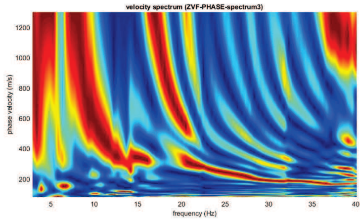
Figura 49: Spetto di velocità, Dataset Onde Rayleigh componente verticale (ZVF)
