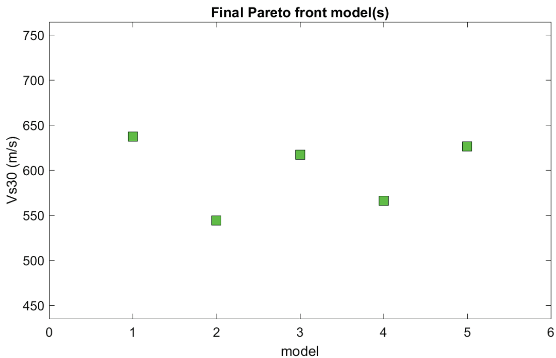
Figura 72: Distribuzione pareto Vs 30
