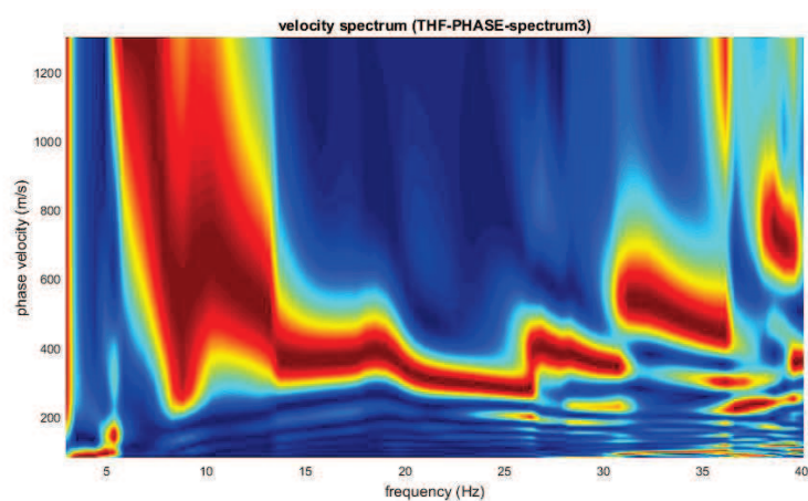
Figura 22: Spetto di velocità, Dataset Onde Love componente orizzontale (THF)
