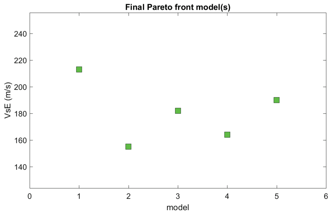
Figura 73: Distribuzione pareto VsE
