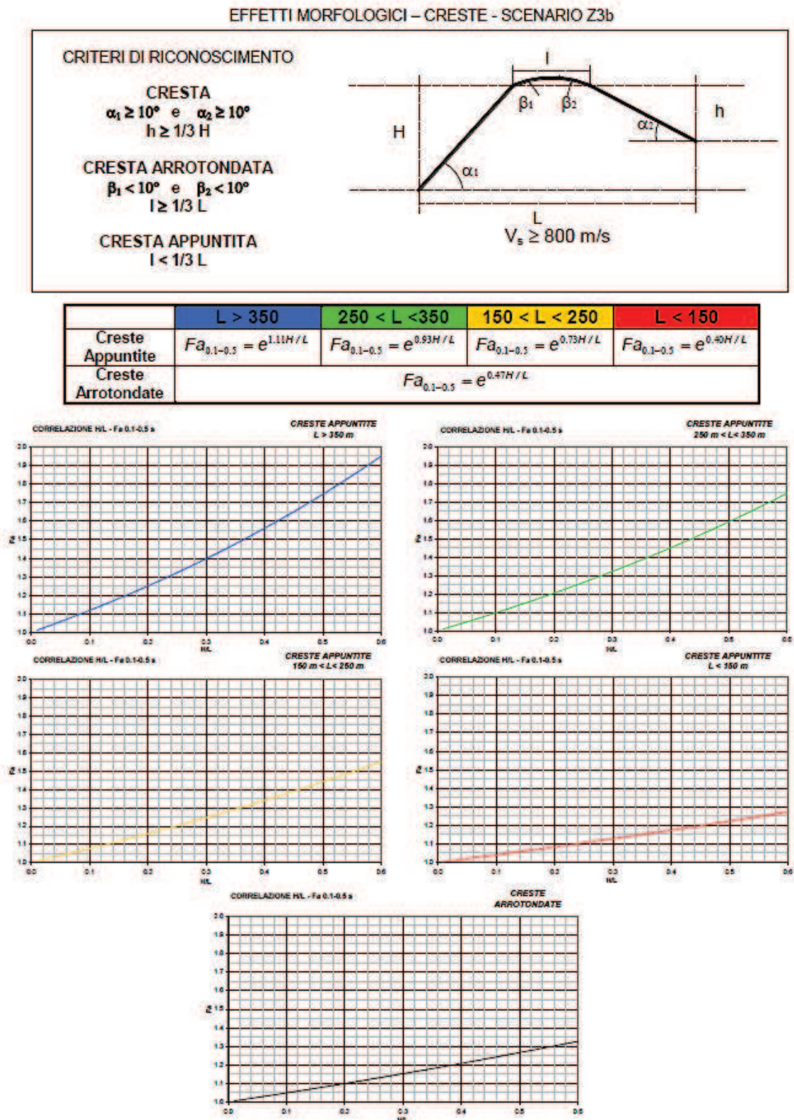
Figura 12: Schema regionale per gli effetti morfologici dello scenario Z3b
