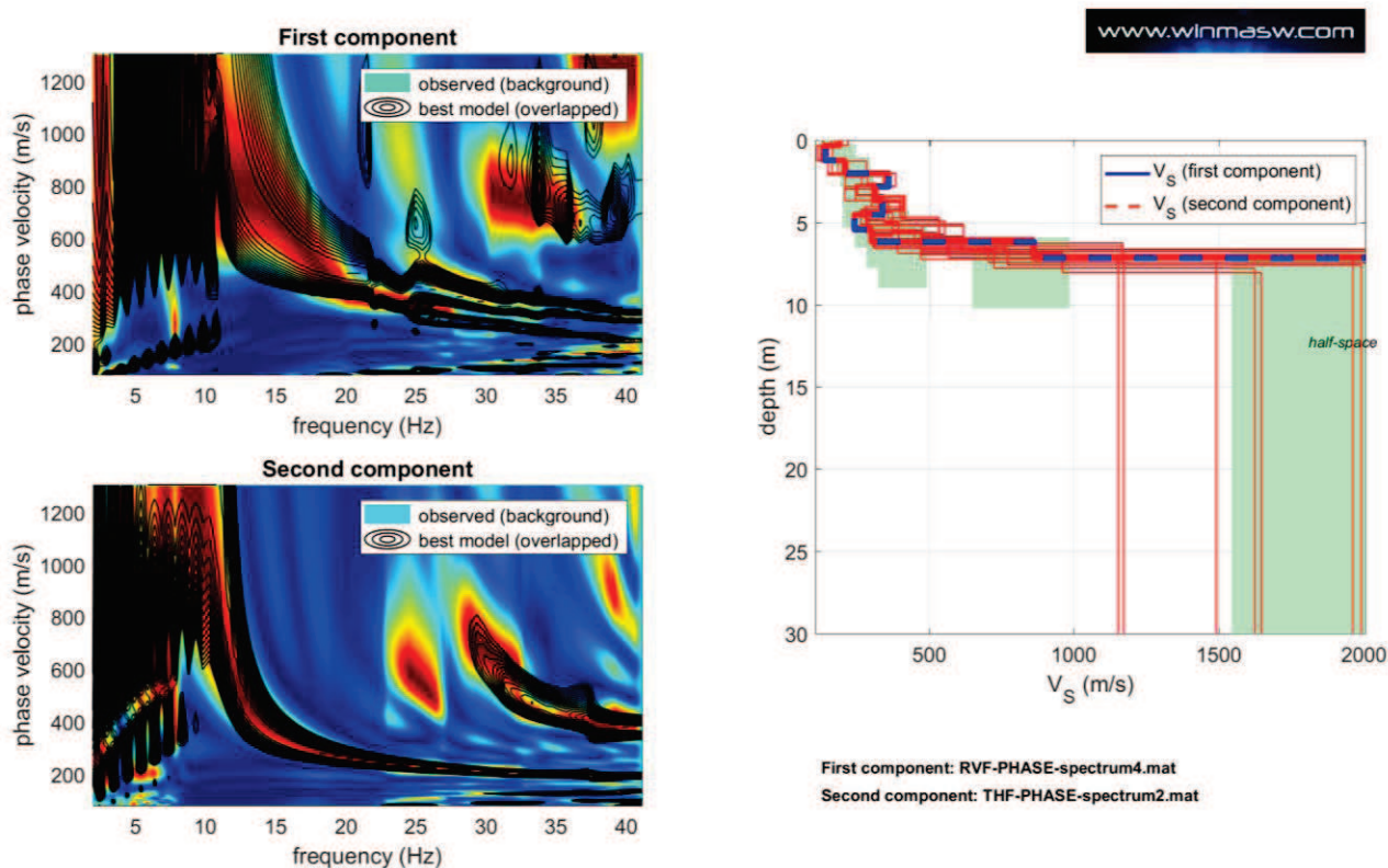
Figura 54: Inversione congiunta Full velocity spectral Rayleigh e Love
