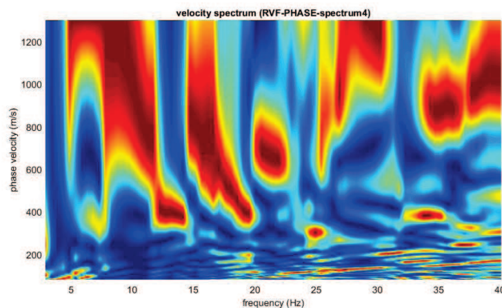
Figura 65: Spetto di velocità, Dataset Onde Rayleigh componente radiale (RVF)
