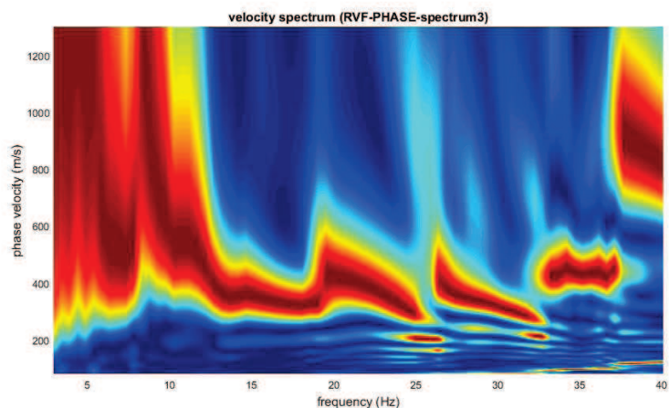
Figura 21: Spetto di velocità, Dataset Onde Rayleigh componente radiale (RVF)
