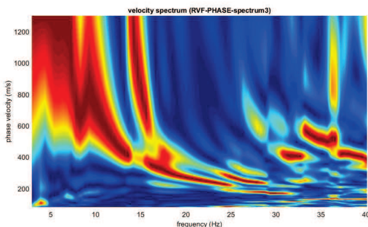
Figura 35: Spetto di velocità, Dataset Onde Rayleigh componente radiale (RVF)
