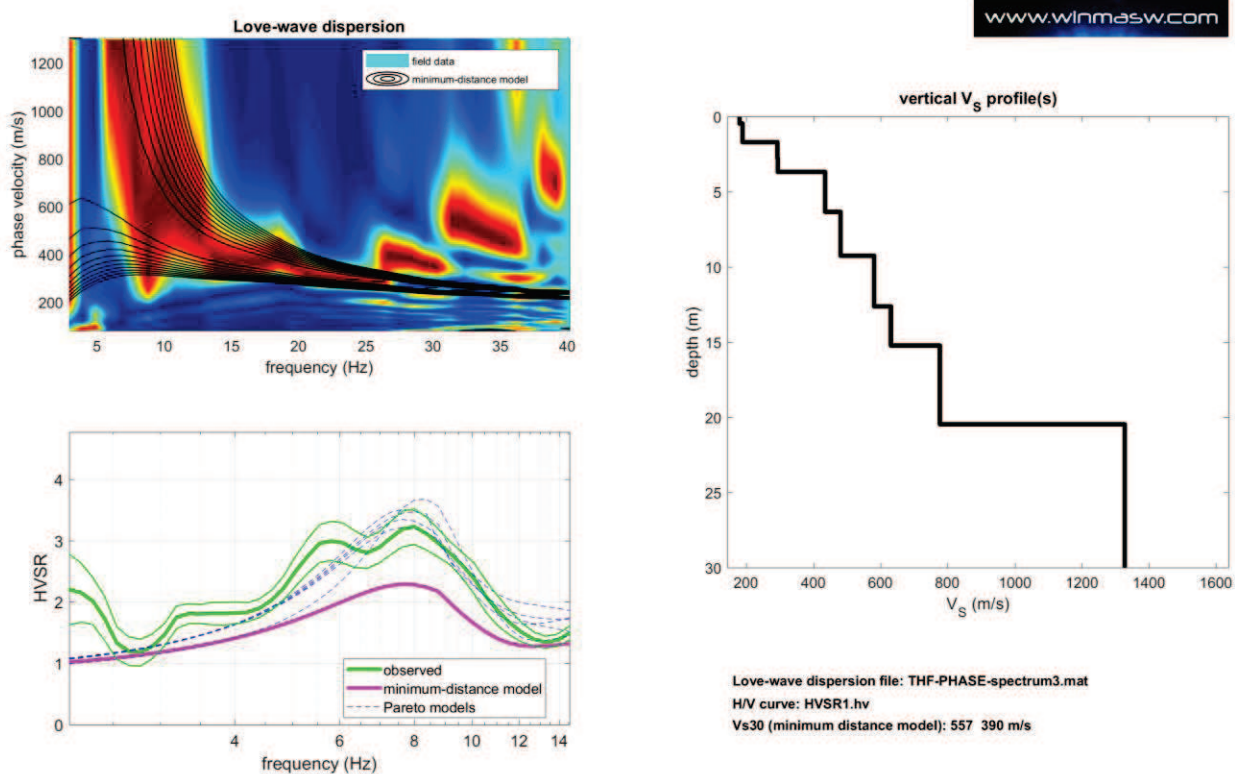
Figura 25: Analisi congiunta onde Love e HVS2 1
