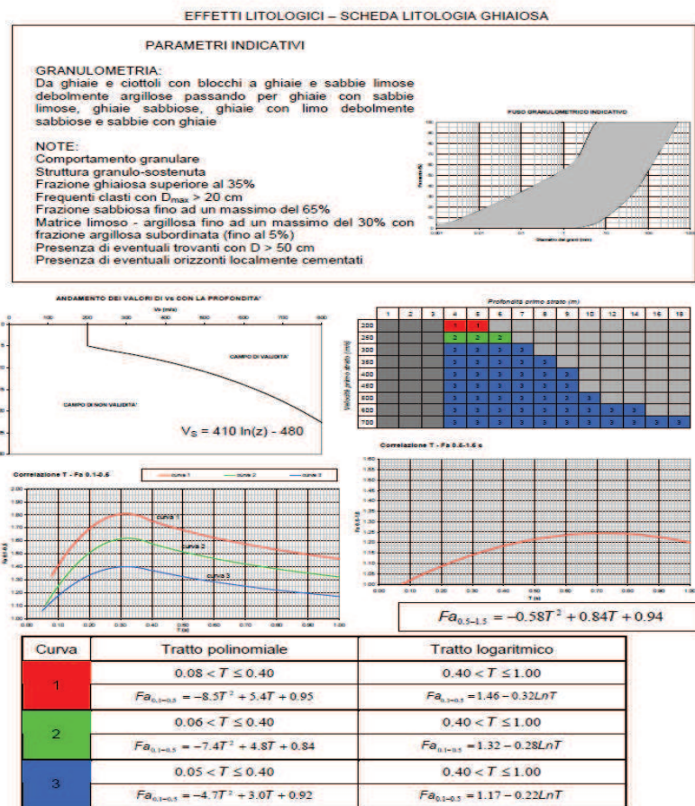
Figura 47: Scheda litologia ghiaiosa
