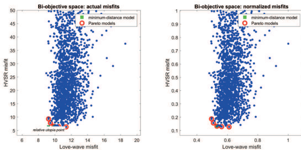
Figura 27: Grafico tra errore HVSR e Love, attuale e normalizzato
