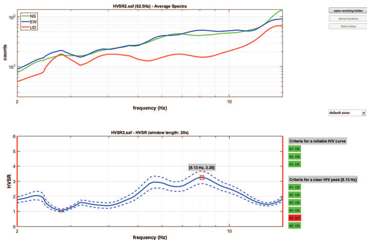
Figura 24: Dati HVS2, nella misura 2 a 8.13 Hz è stato individuato un picco di 3.26 Nella colonna di destra possiamo vedere la verifica dei criteri di ammissibilità del progetto SESAME
