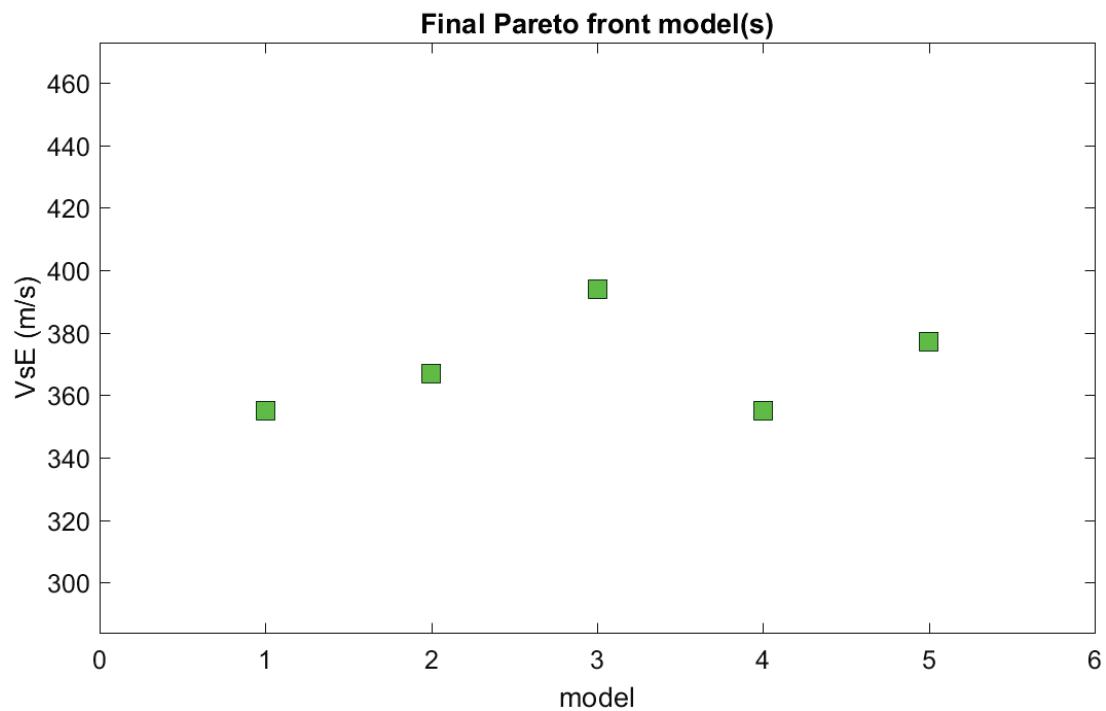
Figura 29: Distribuzione pareto VsE
