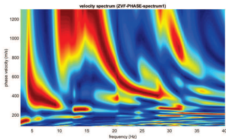
Figura 64: Spetto di velocità, Dataset Onde Rayleigh componente verticale (ZVF)
