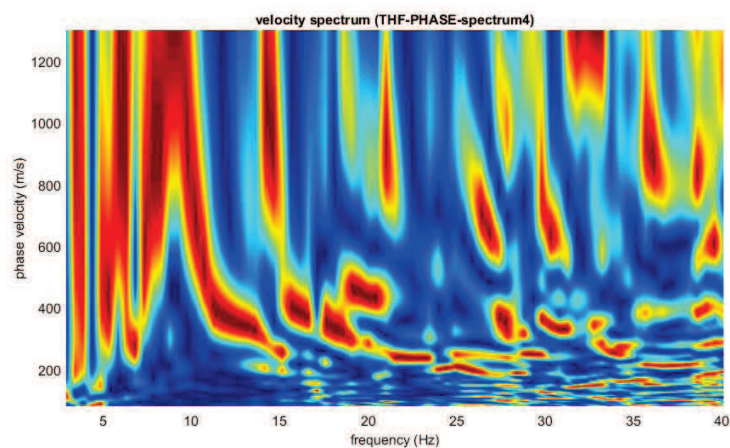
Figura 66: Spetto di velocità, Dataset Onde Love componente orizzontale (THF)
