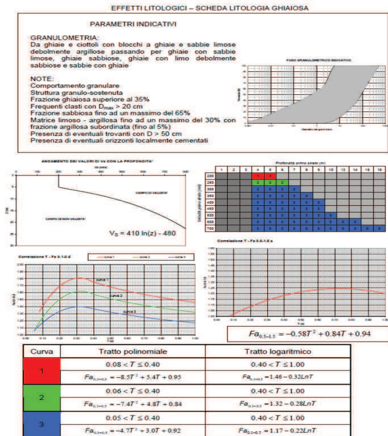
Figura 62: Scheda litologia ghiaiosa
