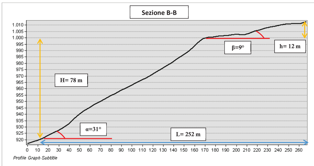
Figura 8: Ubicazione e sezione BB per scenario Z3a
