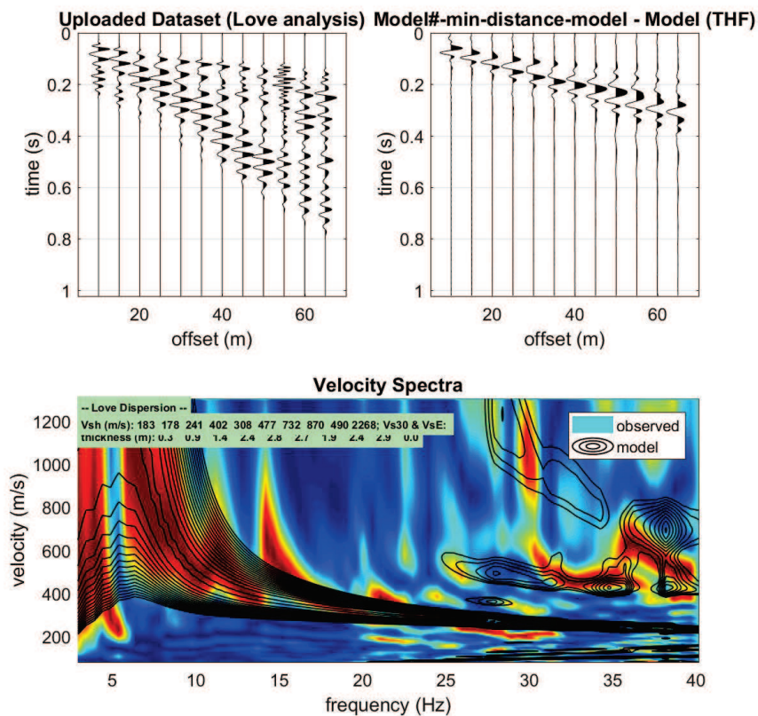
Figura 41: Modello distanza minima in full velocity spectral per le onde di Love
